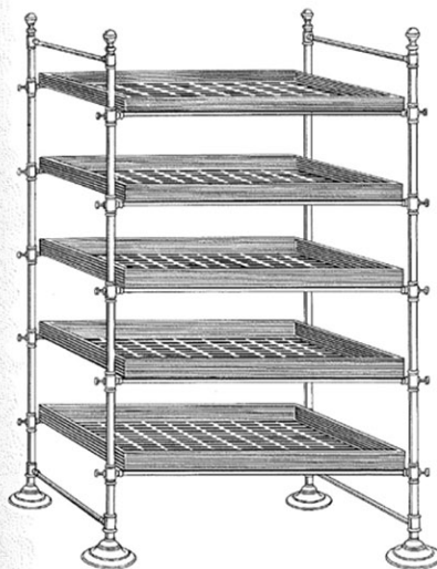
Brödställ Litt. L.
