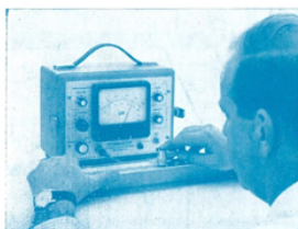
My-mätare för kontroll av eloxeringsskiktets tjocklek.
